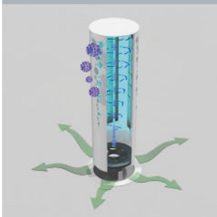
Luft wird im oberen Teil der Säule angesaugt, an UVC-Strahlern entkeimt und unten gereinigt ausgeblasen.
